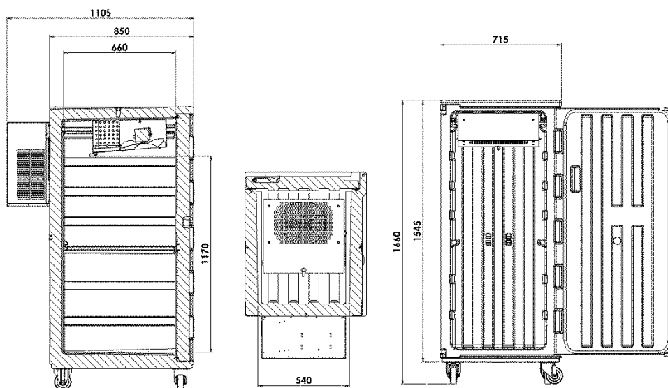
Модель с холод. агрегатом сзади, вент. Арт.: 05009081, 05009083
