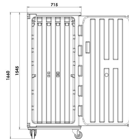
Модель с холод. агрегатом сзади, вент. Арт.: 05009042, 05009082
