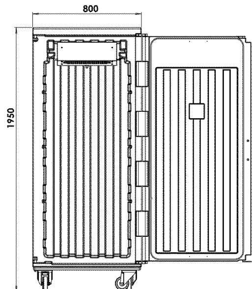
Модель с холод. агрегатом сзади, вент. Арт.: 07809008, 07809011, 07809012, 07809013
