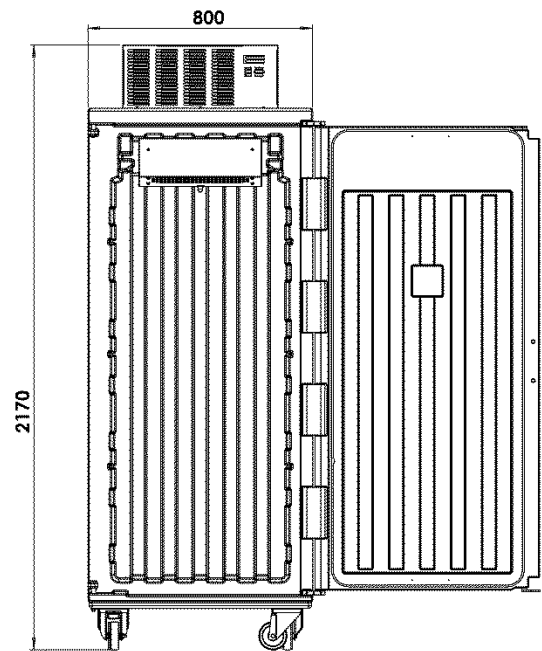
Модель с холод. агрегатом сверху, вент. Арт.: 07809014, 07809015, 07809016, 07809017
